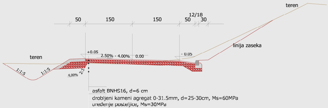
Presek I-I
